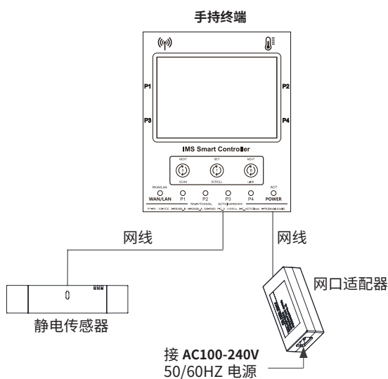
图 14 联接监测终端示意图
