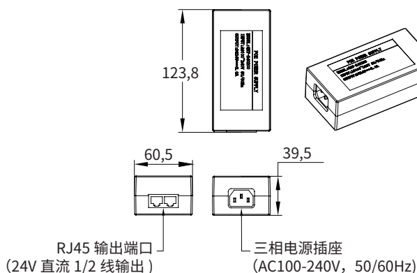
图 5 适配电源外形尺寸图
