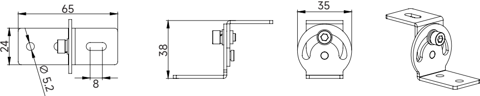
安装挂角外形尺寸图 (选配件)
