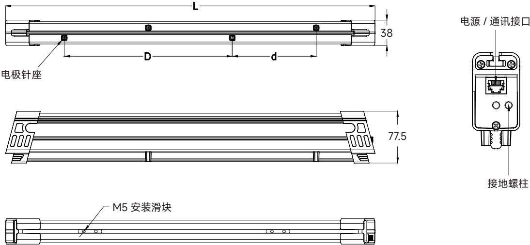
离子棒外形尺寸图
