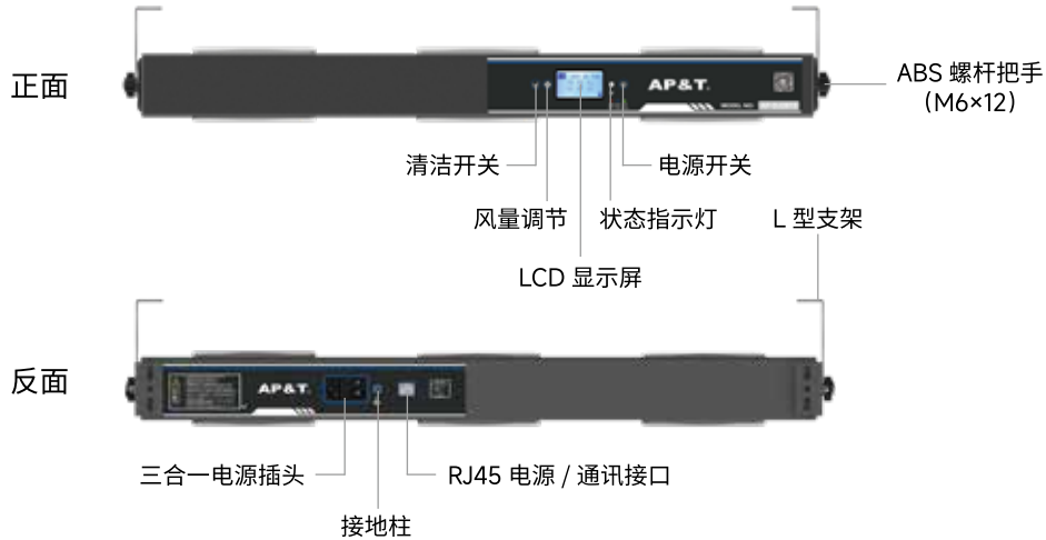
液晶屏参数显示说明
