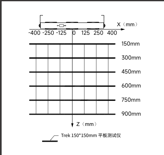
风机测试方位图
