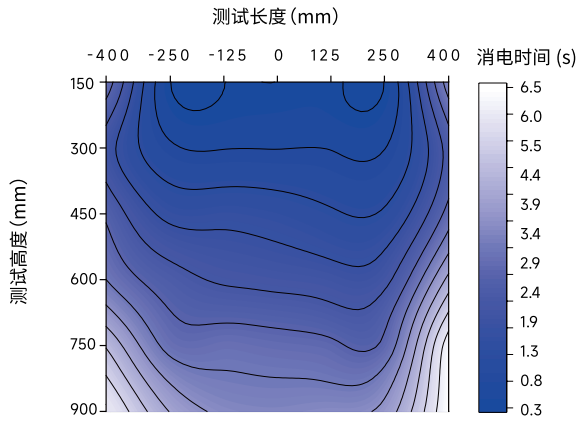
AP-DJ2813 消电时间空间分布图
