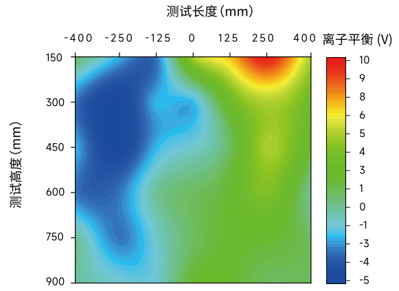
AP-DJ2813 离子平衡空间分布图
