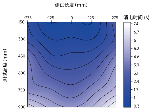
AP-DJ2812 消电时间空间分布图
