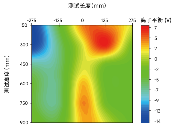
AP-DJ2812 离子平衡空间分布图
