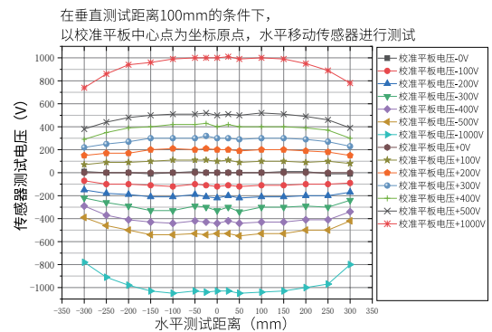
图 4-2 垂直距离 100mm 时，标准平板电极水平测试数据图
